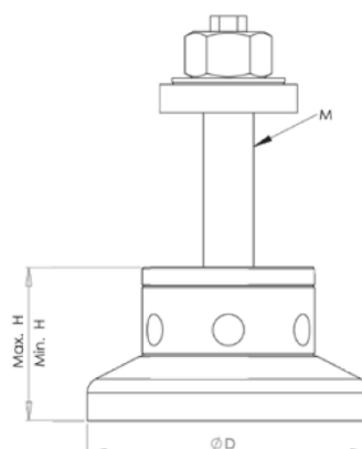
ALS2 con perno de anclaje ZKA
