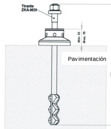
ALS2 con perno de anclaje ZKA
