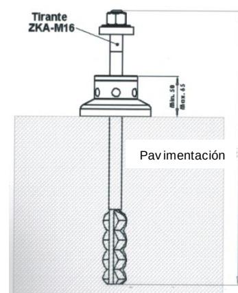
ALS1 con perno de anclaje ZKA
