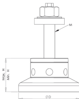
ALS1 con perno de anclaje ZKA
